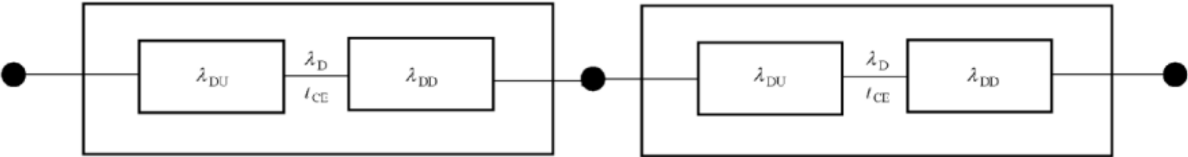
图 B.9 2002 可靠性框图
